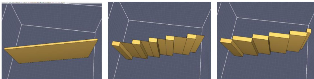
1. sz. ábra. Építményszerkezet ábrázolása a geometria modellben (a), illetve kétféle konvertálási lehetősége (b,c) a cellahálózathoz megfelelően.
