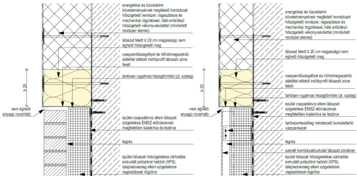
M3 ábra Csomópont javasolt elvi kialakítása légrésees lábazatok esetében
