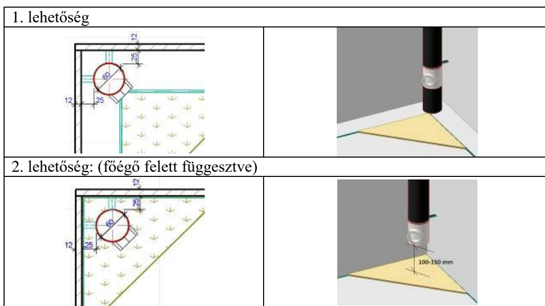
1. táblázat: Kéménycsövek SBI mintájának lehetséges elrendezései
