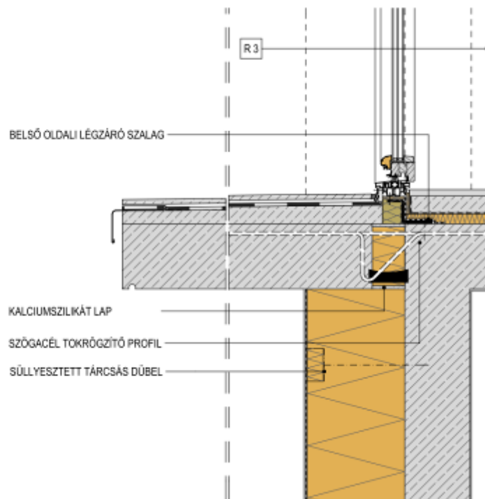
E7 sz. ábra. Erkélykonzol teherbíró elválasztása hőhídmegszakító elemmel
