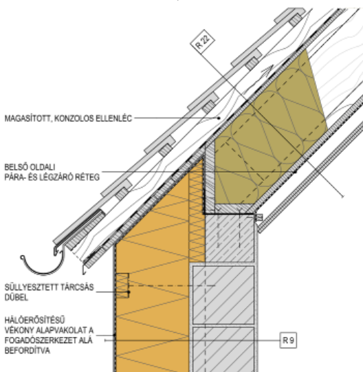
E2 sz. ábra. Falazott, éghető hőszigeteléssel ellátott fal
